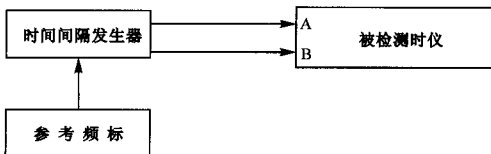
(b) 双脉冲测量
