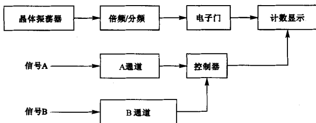
图 1 数字式时间间隔测量仪工作原理图
