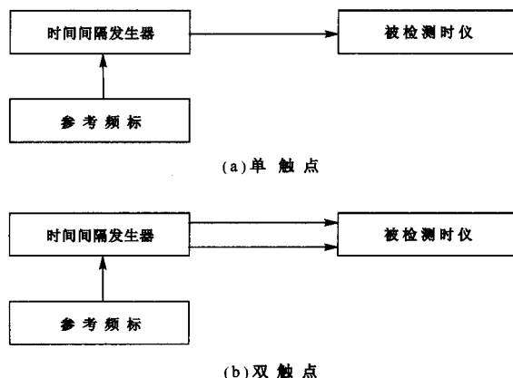
图 4 机械触点动作时间测量的仪器连接图
