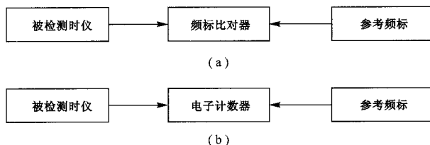
图 2 内部晶振检定的仪器连接图
